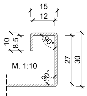
Serie 1 Dreier-Regelkantung
