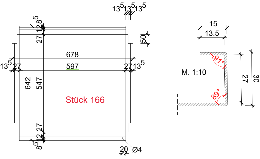
Serie 1 Zweier-Regelkantung
